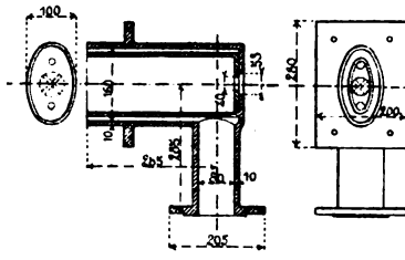
Fig. 34. — Buse pour l'entrée du gaz.
